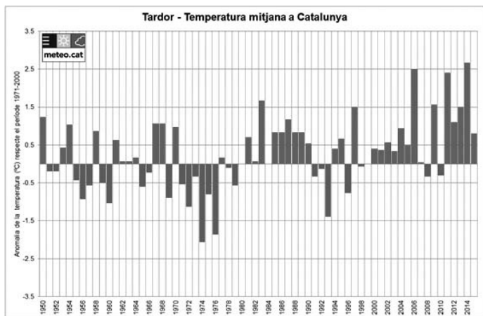
Gràfica 3: Temperatura mitjana de tardor a Catalunya (1950-2015) expressada com a diferència respecte de la mitjana climàtica 1971-2000.
