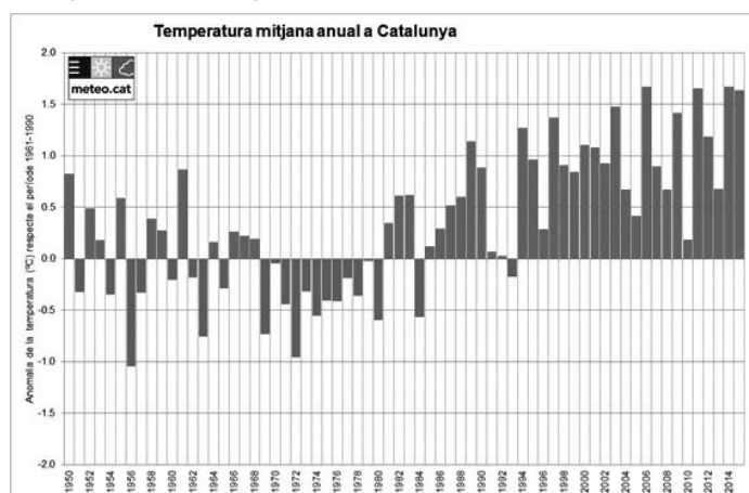
Gràfica 1. Temperatura mitjana anual a Catalunya, expressada com a anomalia respecte a la mitjana 1961-1990
