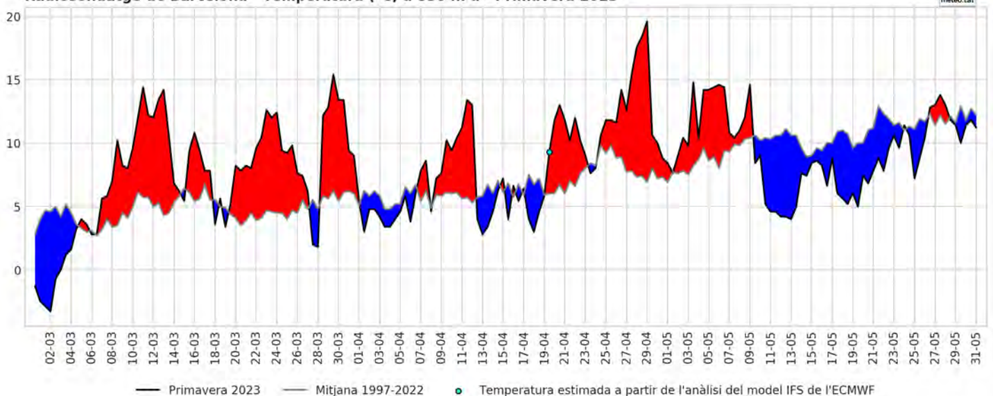
Radiosondatge de Barcelona - Temperatura (°C) a 850 hPa - Primavera 2023
