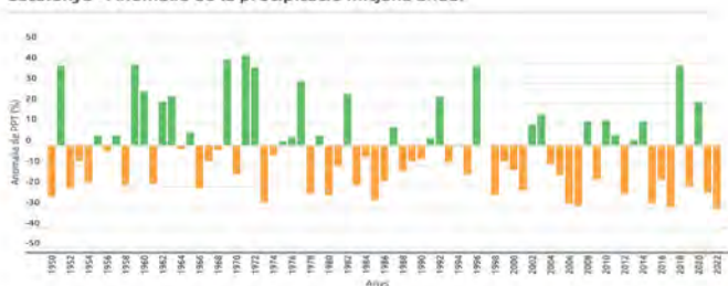
Catalunya - Anomalia de la precipitació mitjana anual
